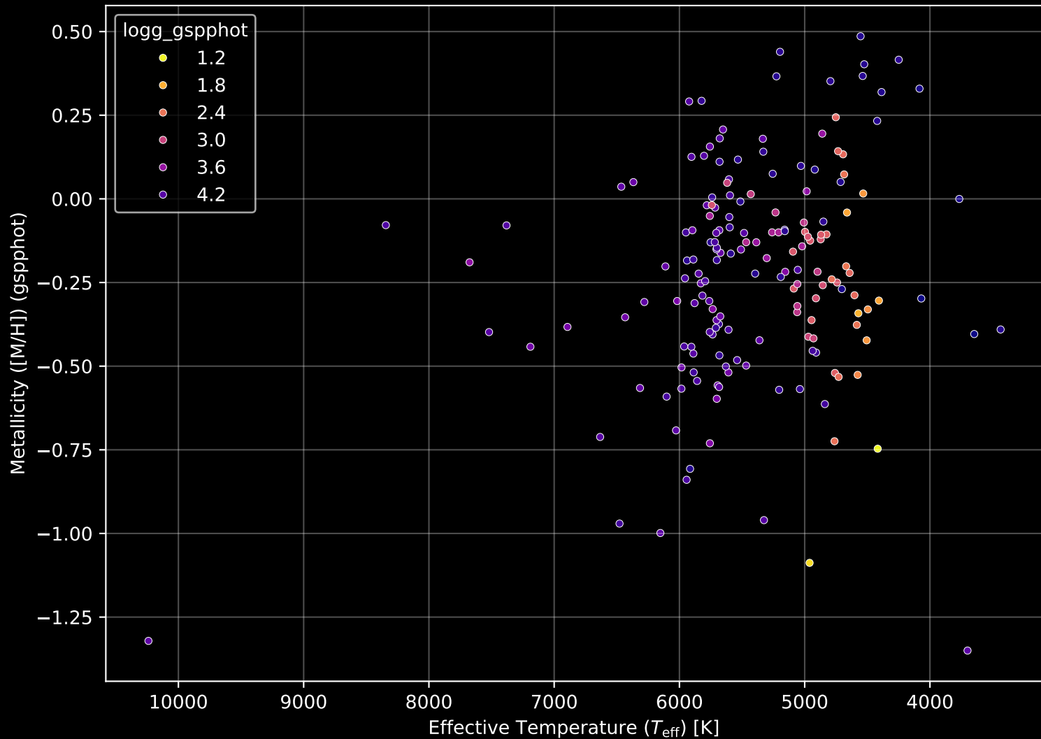
APOGEE DR17 Field: [264-26-O_TESS] Stellar Population Parameters (n= 173)
